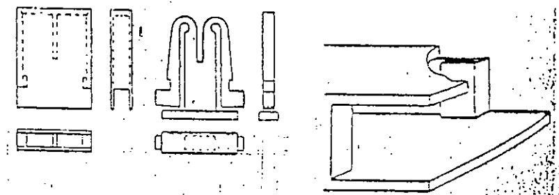
Cierre de trinquete, hoja con embujadores a los costados
