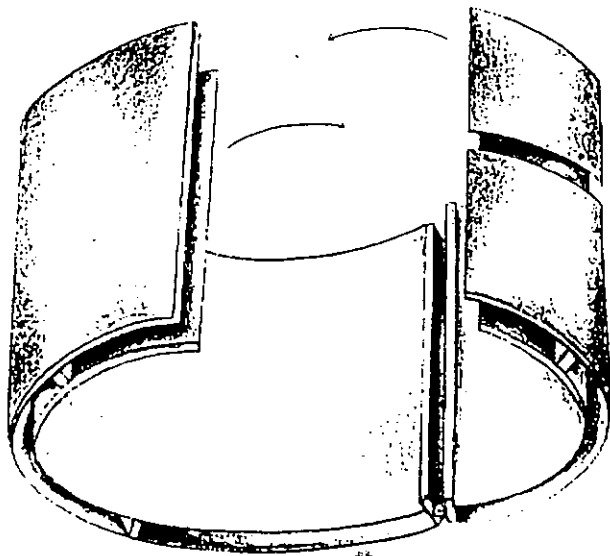
Mecanismo de Apertura y Cierre
