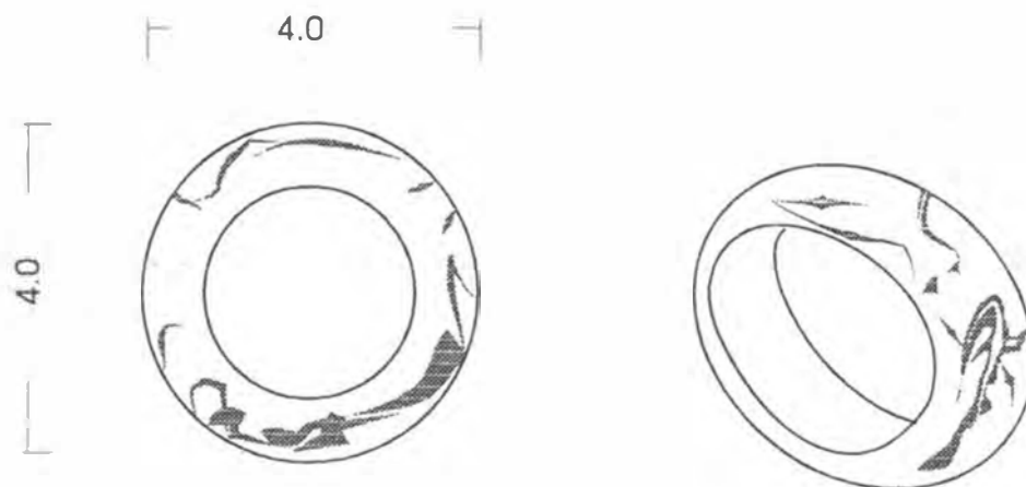
VISTA SUPERIOR
