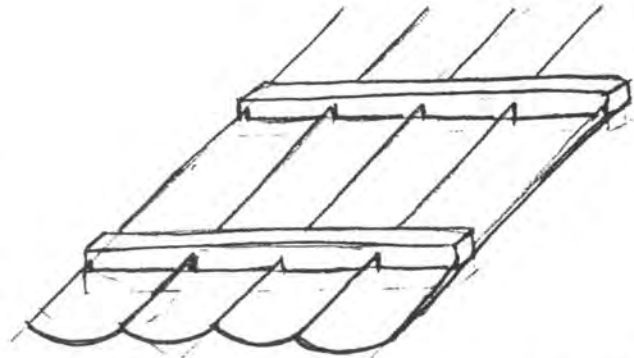
DETALLE DE ESTRUCTURA PARA UNIR LA GUADUA
