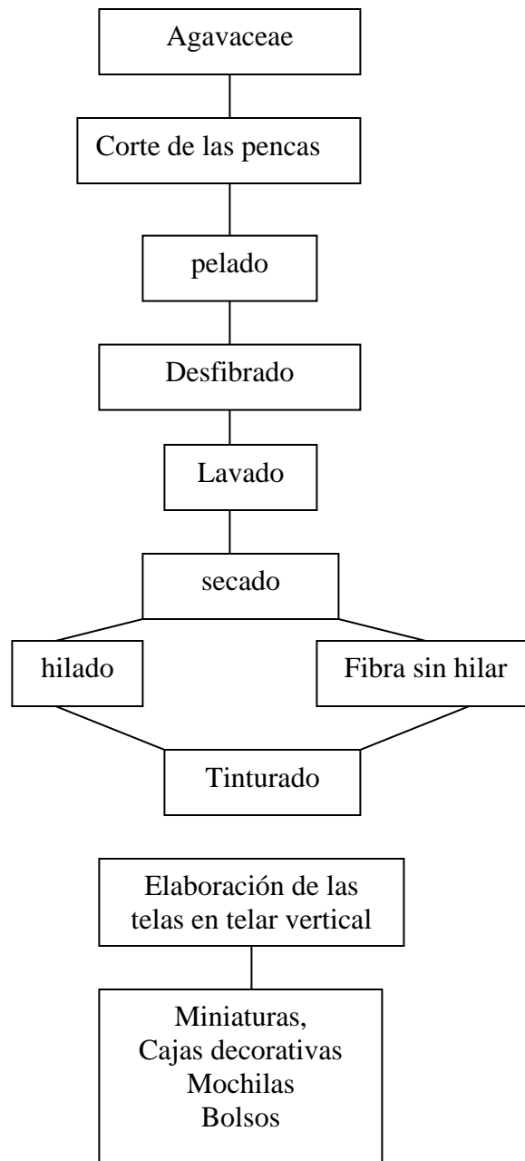
Diagrama de proceso de producción, materia prima fique
