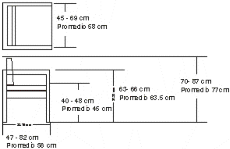
Dimensiones Estandar Silla Aux. con Brazos
