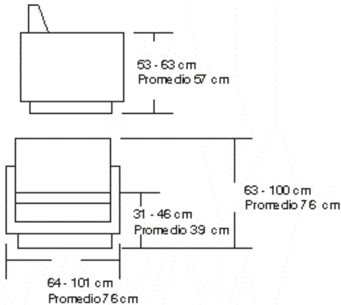
Dimensiones silla Típica de salón
