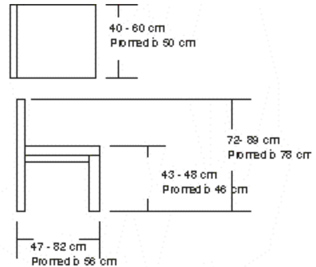
Dimensiones Estandar Silla
