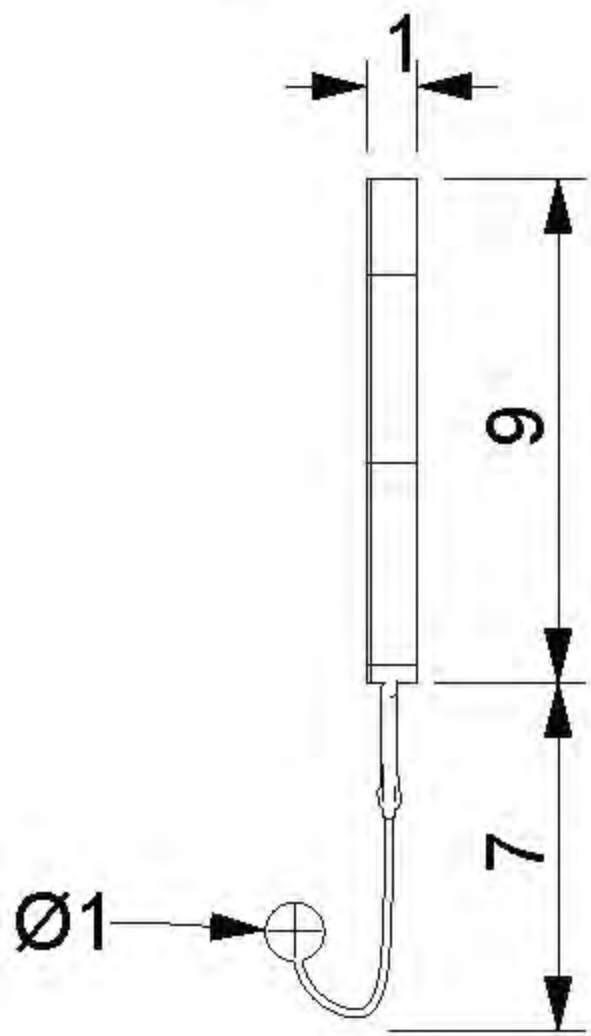
Vista Lateral
