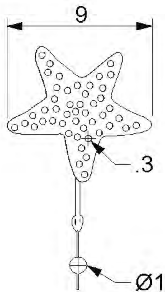
Vista Superior
