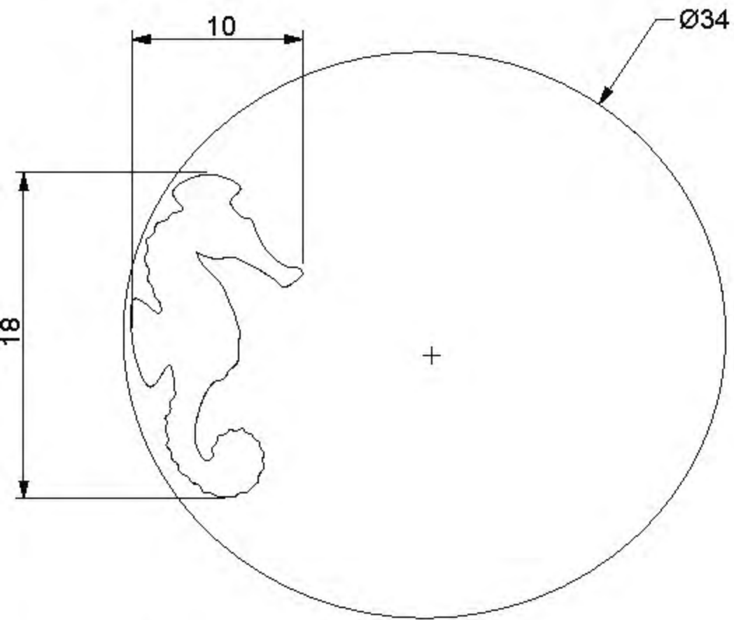
Vista Superior
