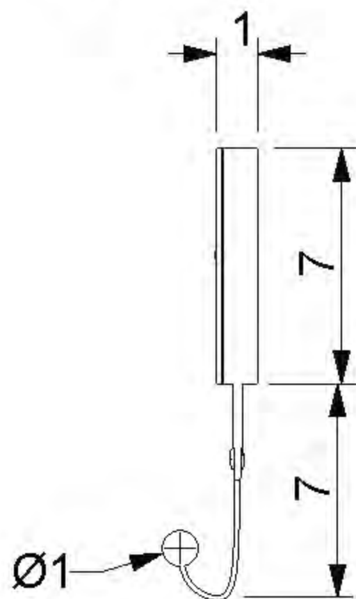
Vista Lateral
