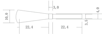
Vista Lateral derecha
