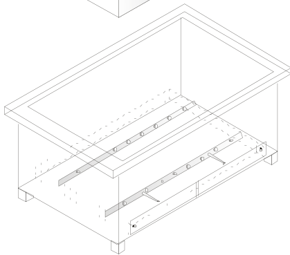
Estufa acero inoxidable con aislante térmico y controles de temperatura y tiempos, y sistema de desagüe
