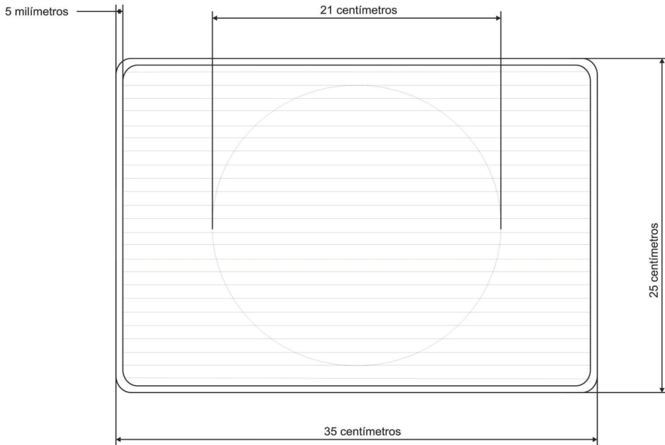
Vista Superior
