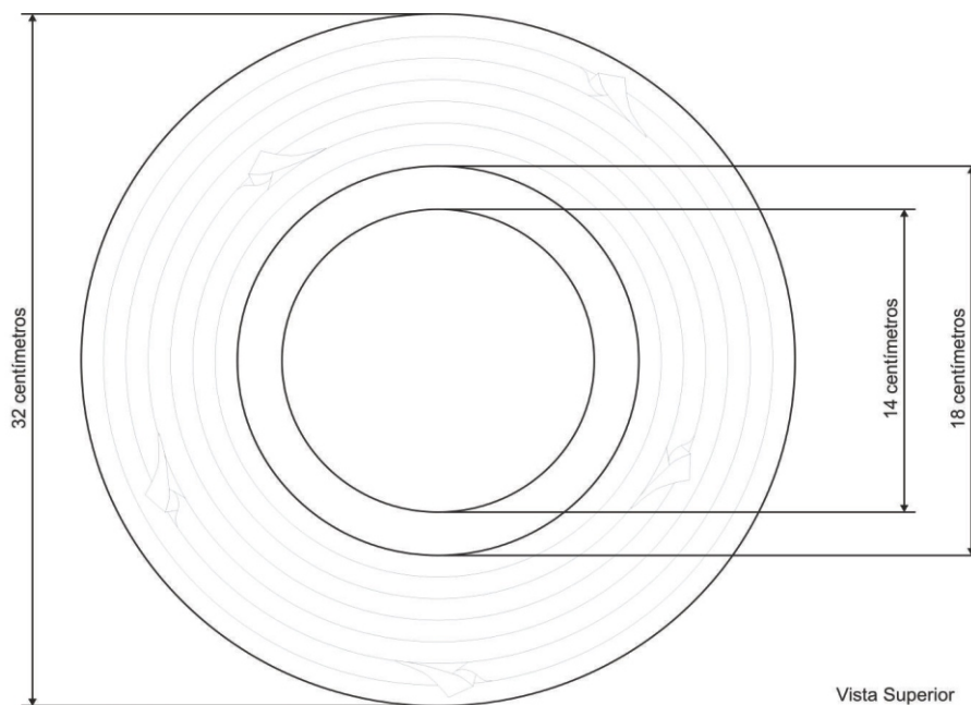
Vista Superior
